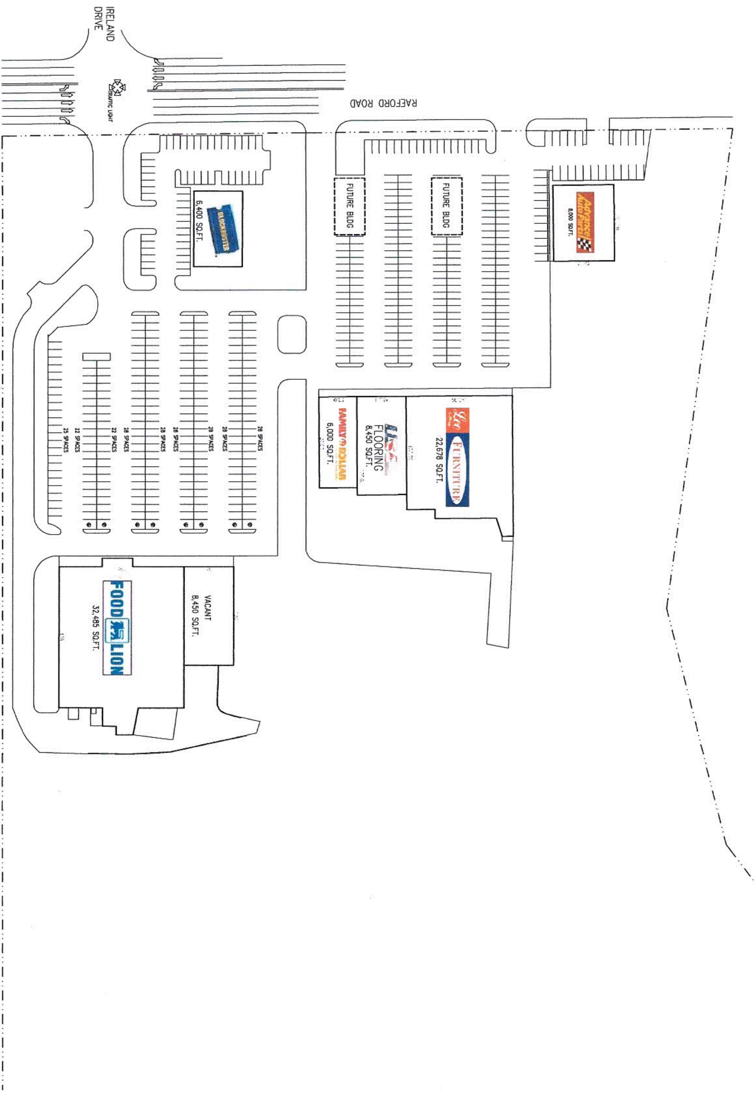
SITEPLAN SCALE: 1" = 50'-0"
